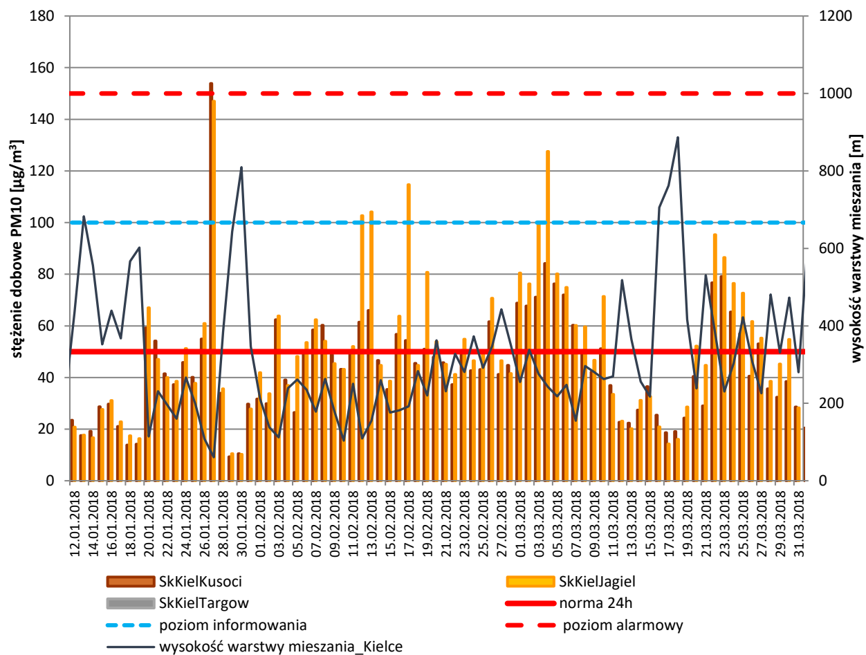
Rysunek 26. Porównanie przebiegu zmienności stężeń 24-godz. PM10 w I kwartale 2018 r. w Kielcach z wysokością warstwy mieszanja
