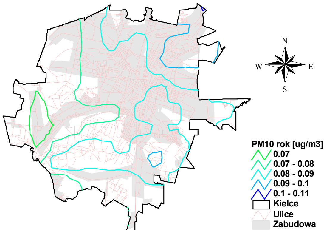
Rysunek 36 Stężenia PM 10 rok w Kielcach pochodzące od emitorów punktowych o h >30m zlokalizowanych na terenie województwa świętokrzyskiego poza pasem 30km wokół Kielc w 2005r.
