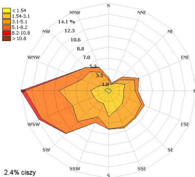
Rysunek 4 Róża wiatrów na stanowisku z modelu UMPL zlokalizowanym w pobliżu miasta Kielce – półroczu zimowe (2005r.)
