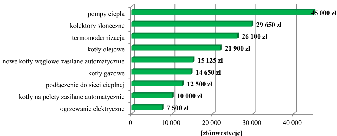
Rysunek 19. Średnie koszty inwestycyjne dla różnych przedsięwzięć związanych ze zmianą sposobu ogrzewania 120
