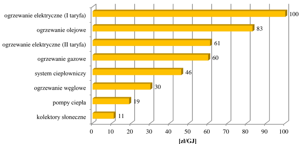
Rysunek 21. Średni koszt uzyskania energii ciepłej 122
