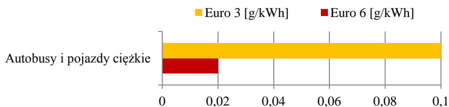
Rysunek 17. Porównanie norm Euro 3 i Euro 6 dotyczących emisji cząstek stałych dla autobusów i pojazdów ciężkich 113
