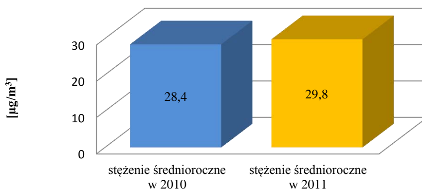
Rysunek 9. Stężenia średnioroczne pyłu zawieszonego PM 2,5 w 2010 oraz 2011 na stacji pomiarowej w miejscowości Busko-Zdrój 96
