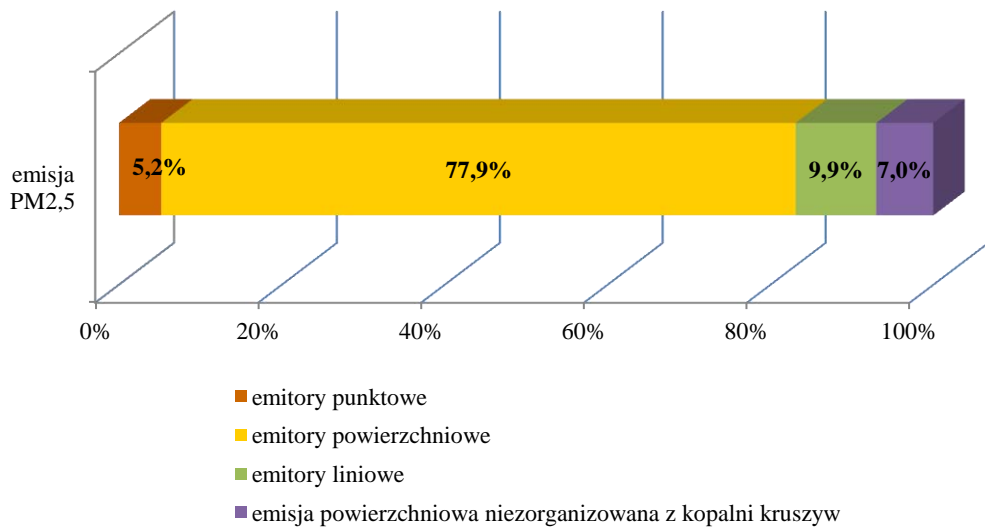
Rysunek 7. Procentowe udziały poszczególnych źródeł emisji w rocznej emisji pyłu PM 2,5 w strefie świętokrzyskiej w 2011 roku 92
