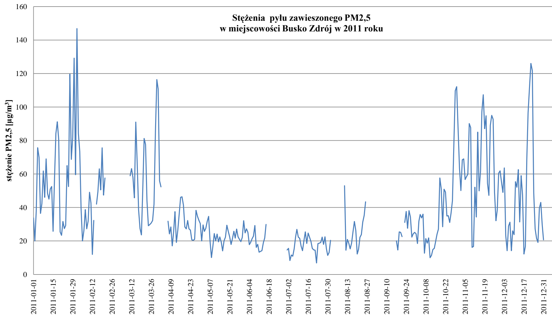
Rysunek 11. Przebieg zmienności stężeń dobowych pyłu zawieszonego PM2,5 w miejscowości Busko-Zdrój w 2011 roku 98
