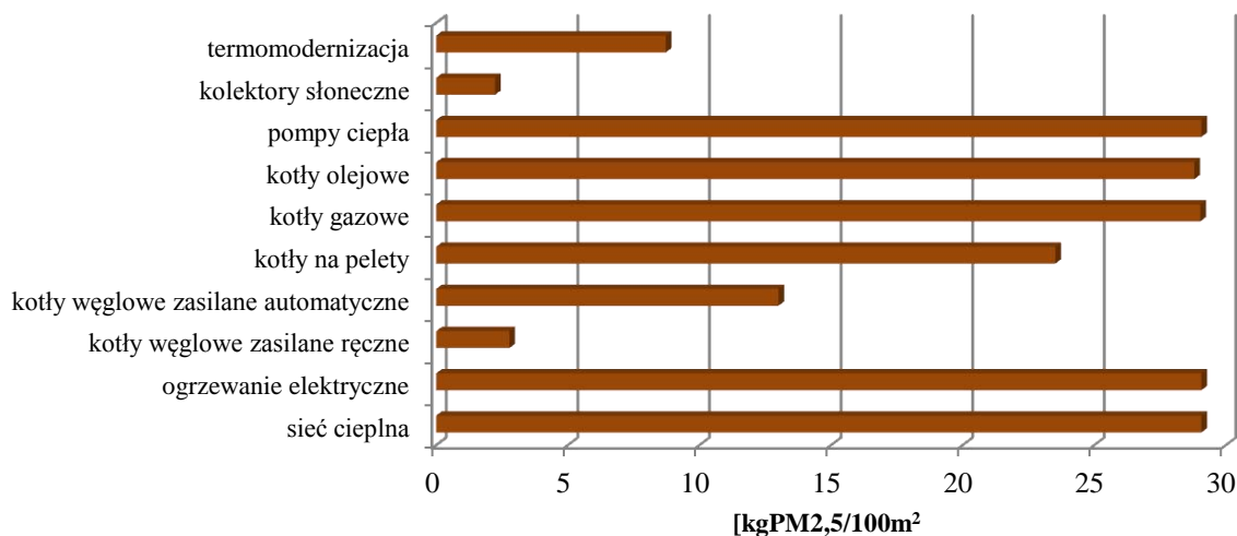
Rysunek 20. Efekt ekologiczny działań/inwestycji w postaci redukcji pyłu PM 2,5 121
