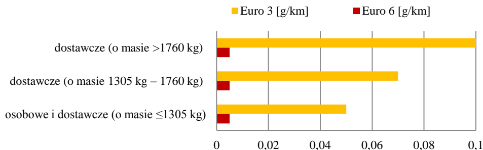
Rysunek 16. Porównanie norm Euro 3 i Euro 6 dotyczących emisji cząstek stałych dla pojazdów osobowych i dostawczych 112
