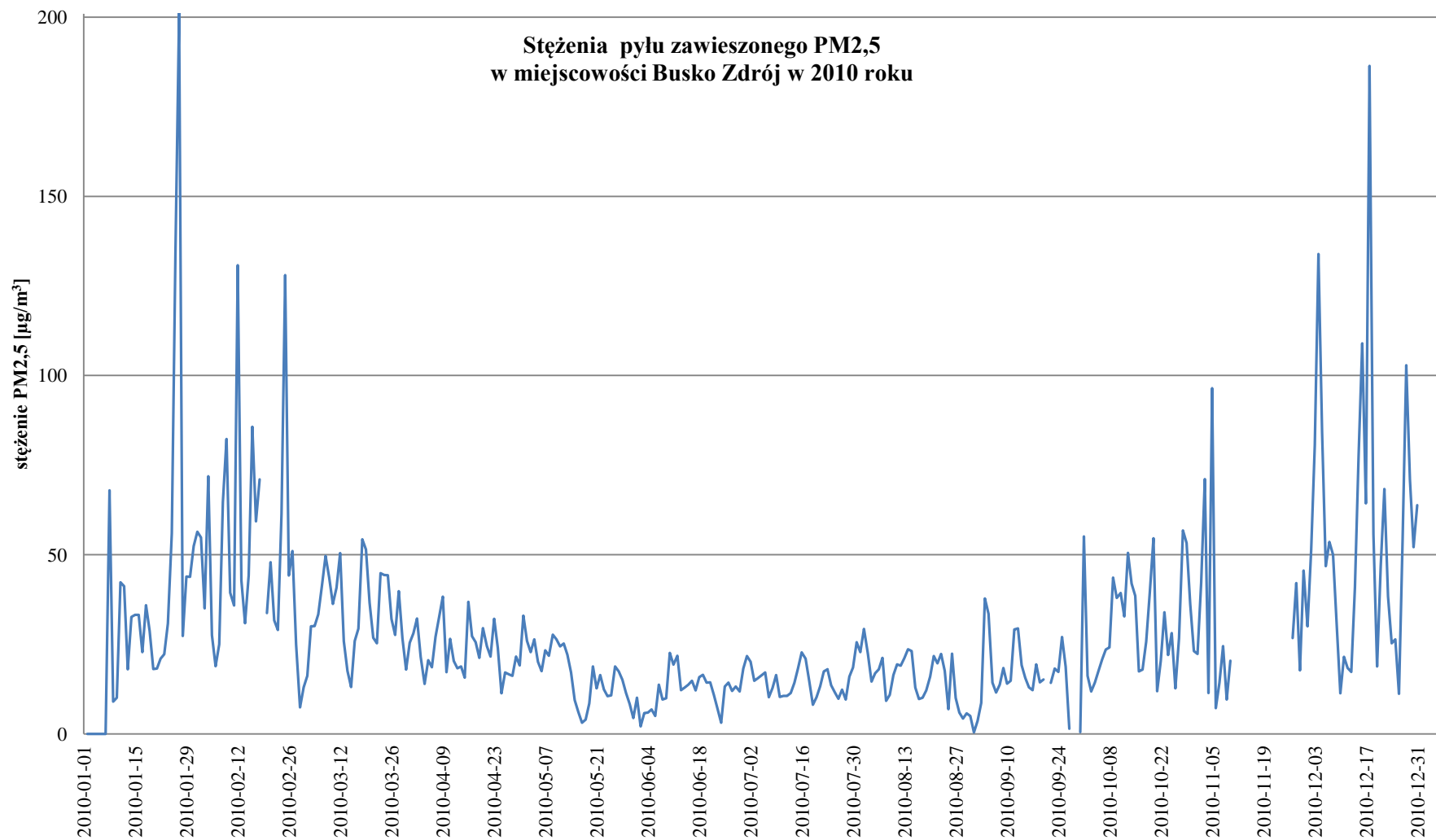
Rysunek 10. Przebieg zmienności stężeń dobowych pyłu zawieszonego PM2,5 w miejscowości Busko-Zdrój w 2010 roku 97
