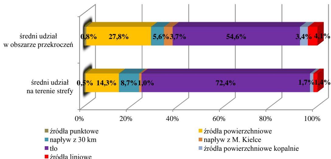
Rysunek 13. Udział poszczególnych źródeł emisji w imisji pyłu zawieszonego PM 2,5 na terenie strefy świętokrzyskiej w 2011 roku 103
