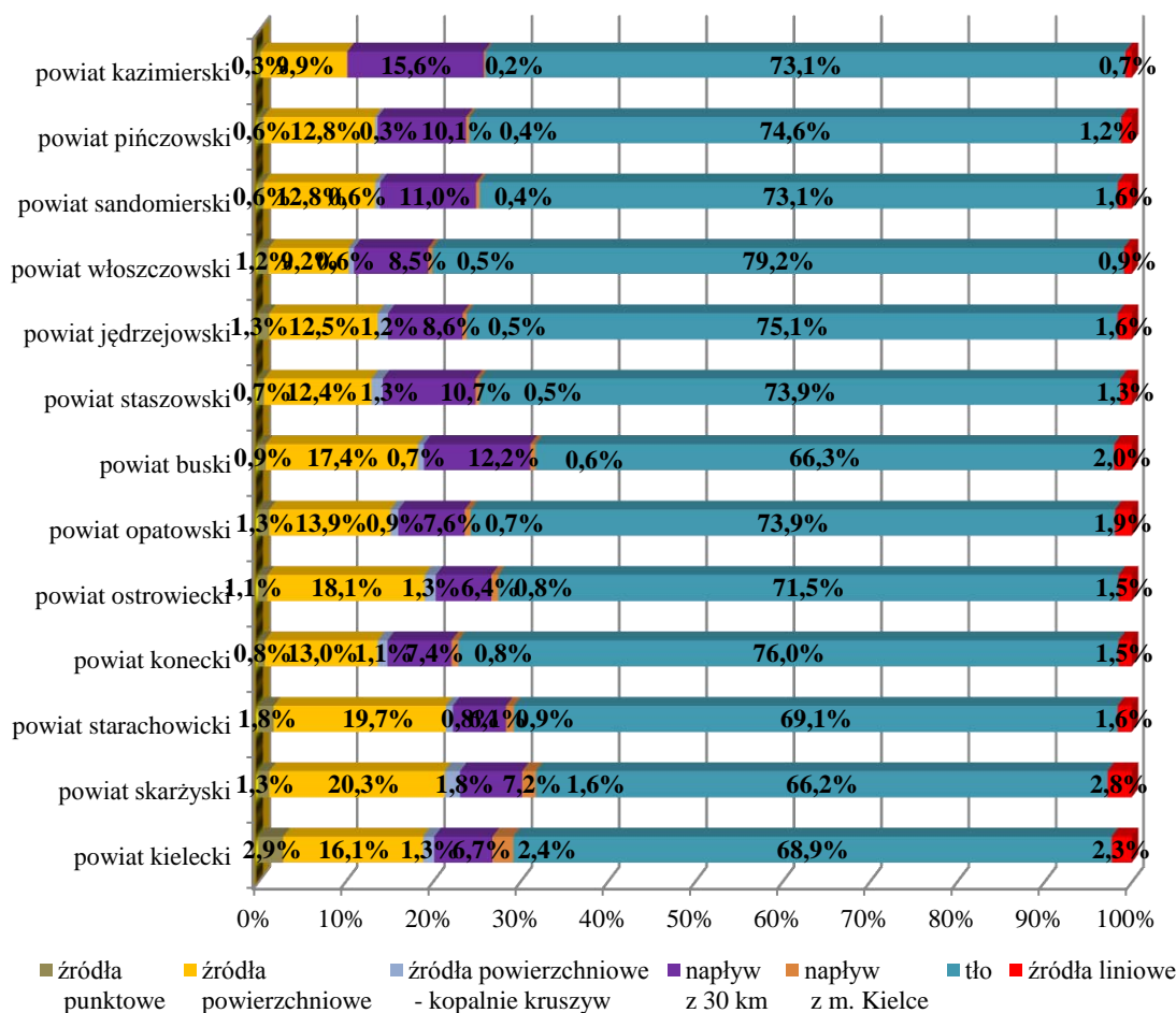
Rysunek 14. Udział poszczególnych źródeł emisji w imisji pyłu zawieszonego PM 2,5 na terenie powiatów strefy świętokrzyskiej w 2011 roku -średnie udziały 105
