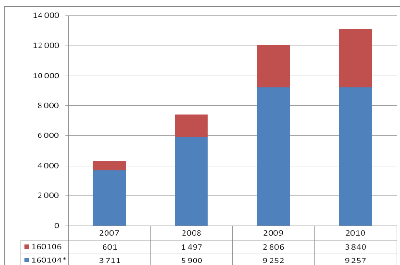
Rysunek 48. Masa zużytych lub nienadających się do użytkowania pojazdów poddanych procesom odzysku (R15) w latach 2007-2010
